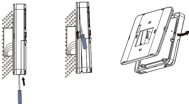
第一步:用平口起撬开前面板
