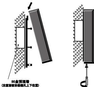
读卡器安装
