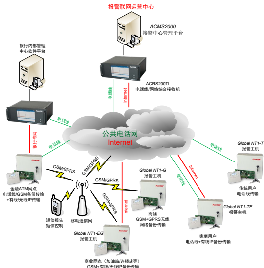
GLOBAL NT1 多网多中心报警联网应用方案
